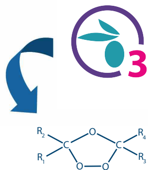
STABILNÍ OZONIDY
